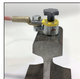
* Aimant applicable au détecteur VTC-OA I
